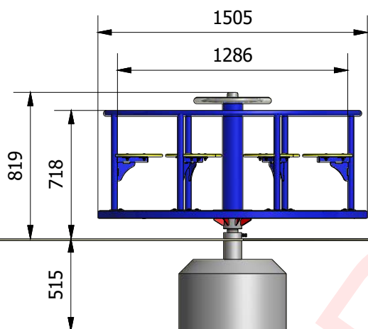
WIDOK 1
